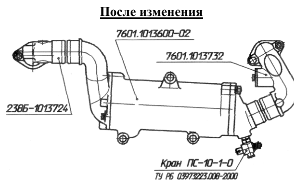
Рис. 2. Теплообменник 7601.1013600-02
