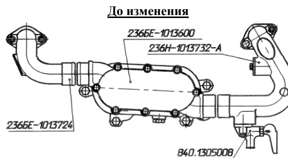
Рис. 3. Теплообменник 236БЕ-1013600
