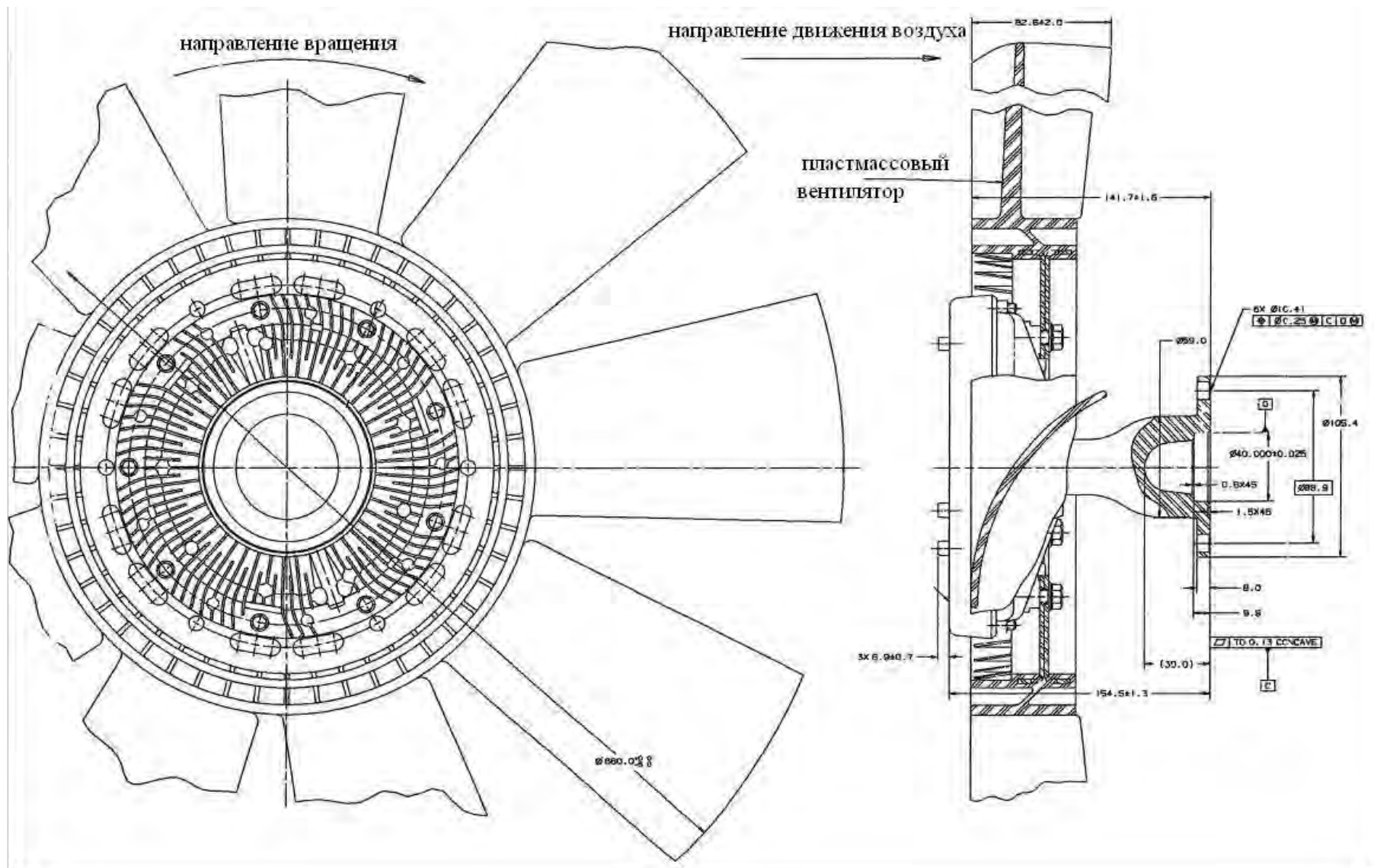
Рисунок 1. Вентилятор "Borg Warner" 020004136.
